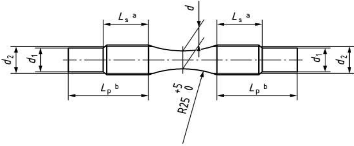
NUMUNE ÖLÇÜLERİ
